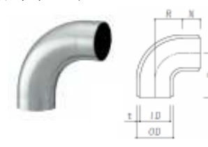
90° ネック付ショートエルボ SGP
